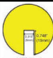
Edge Guard Type B
