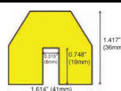
Edge Guard Type BB
