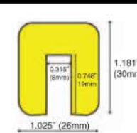
Edge Guard Type G
